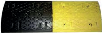
MODELO GO100 AMARILLO / NEGRO MEDIDAS: 100 CMTS LARGO X 32 CMTS ANCHO X 4,5 CMTS ALTO MATERIAL: CAUCHO RECICLADO
